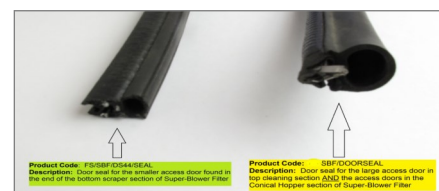
DOOR SEALS
